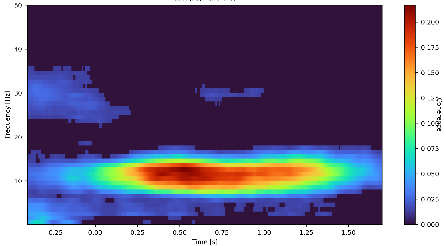
6DR (F2) - 8AD (F6)
